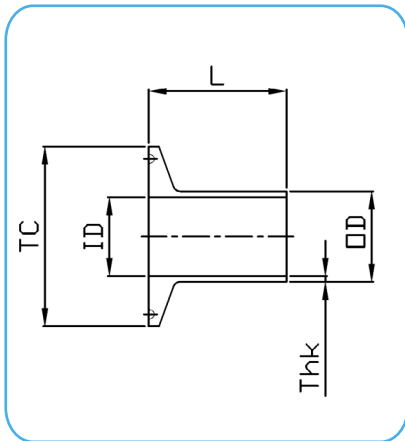
FERRULE CLAMP ASME BPE DT-4.1.4-1
